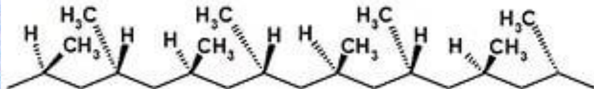
изотактический полипропилен
