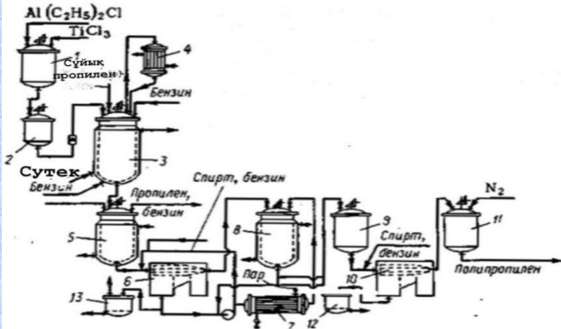
Сурет 1. Полипропилен алу үрдісінің схемасы.
