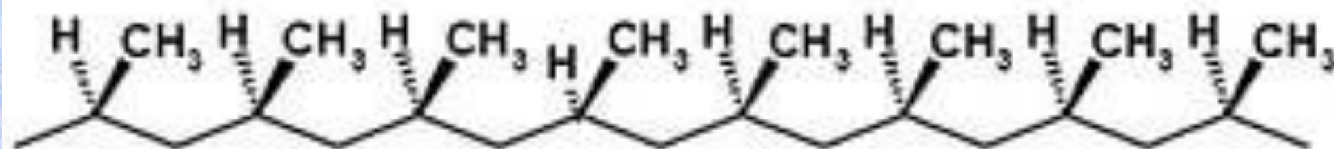
изотактический полипропилен
