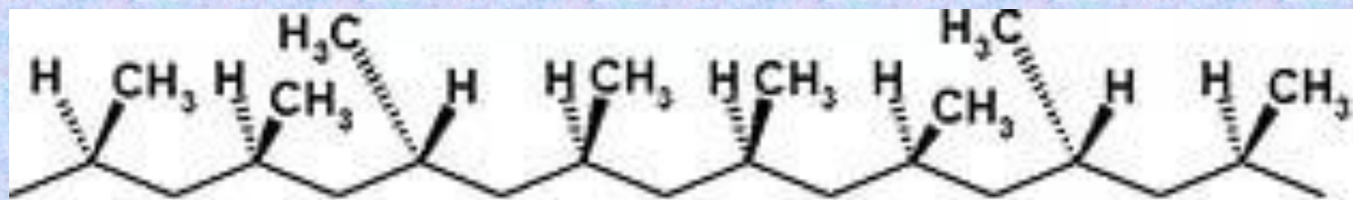
атактический полипропилен
